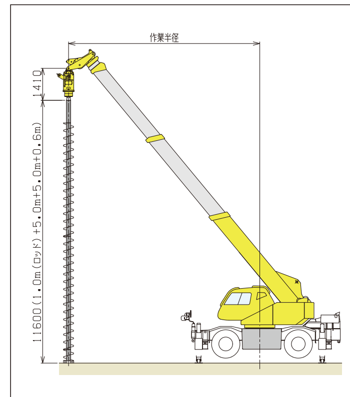
■ 16t・20t 通常作業姿勢
