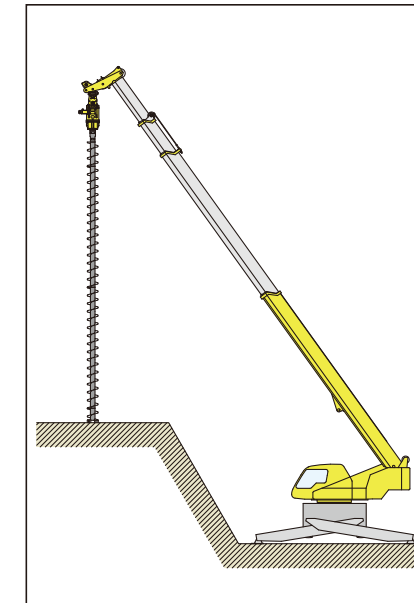
■ 上段差杭打作業
