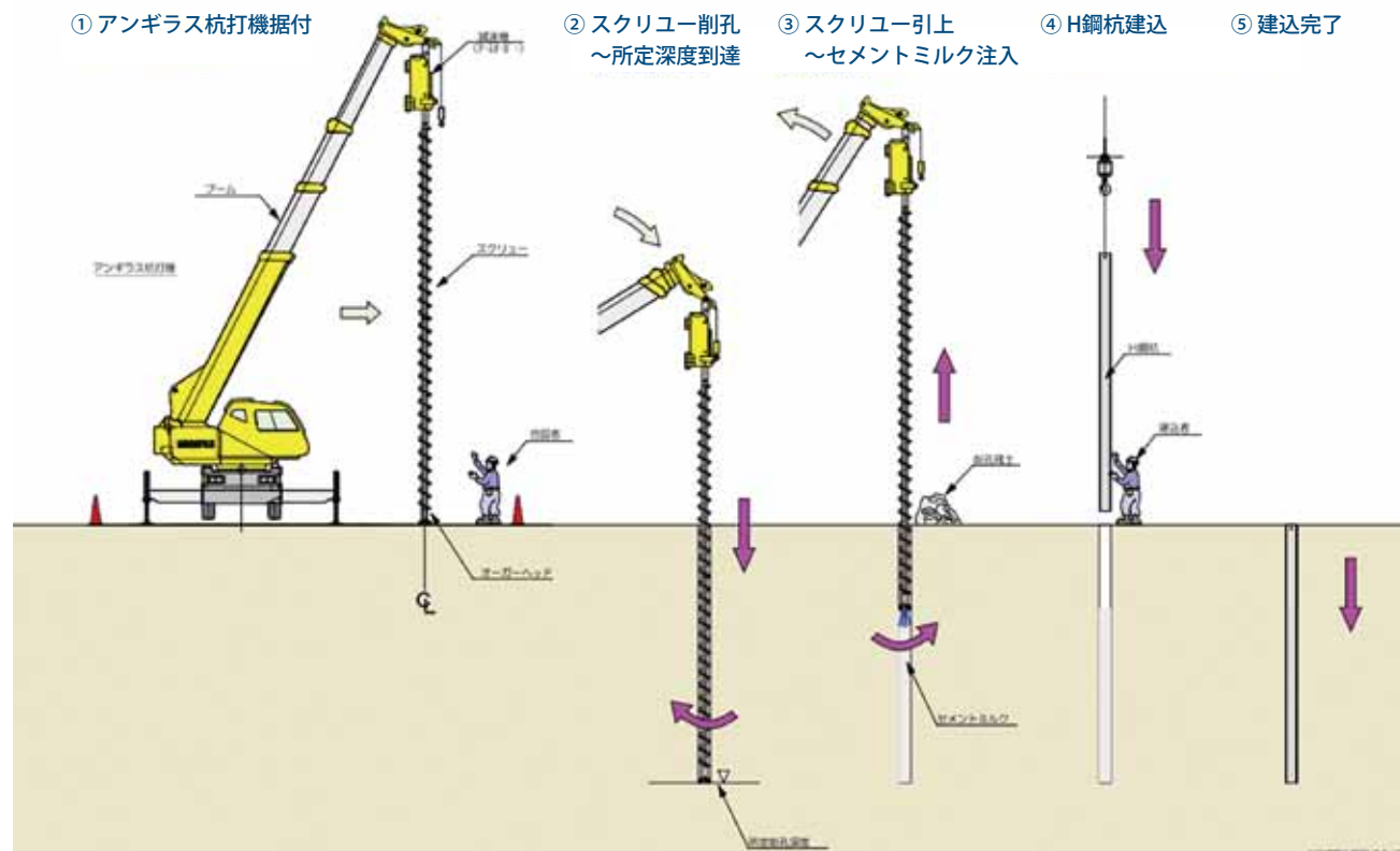
アンギラス杭打機 削孔注入工 施工フロー図
