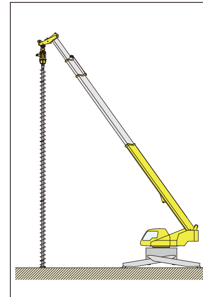
■ 通常フラット盤での杭打作業
