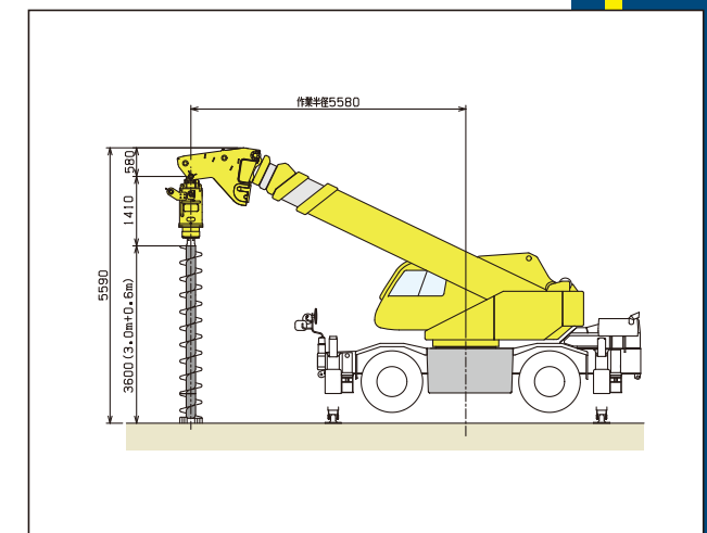
■ 16t・20t 低空頭作業姿勢
